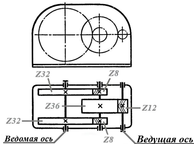
Кинематическая схема
