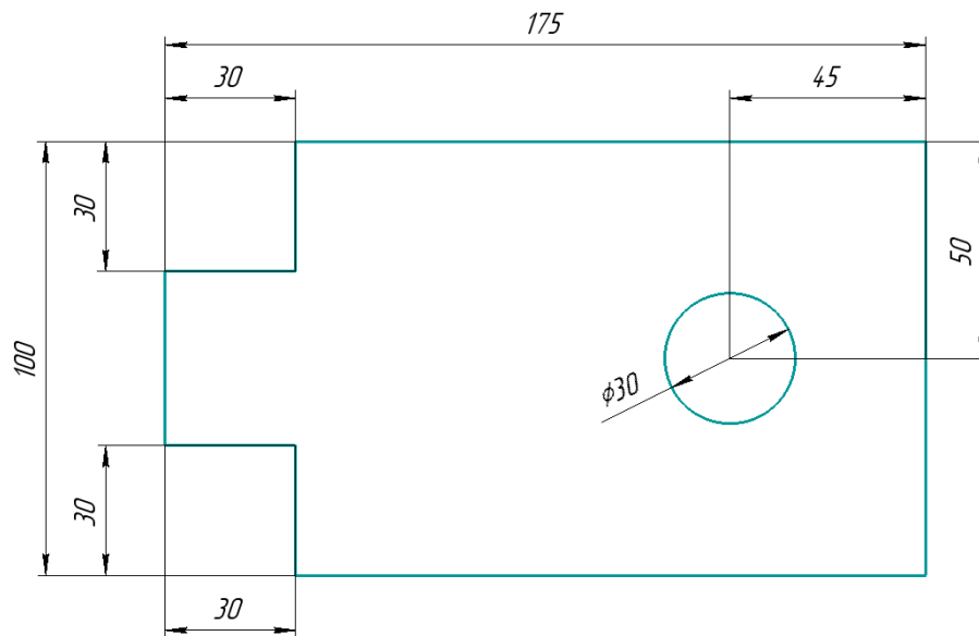
Чертёж детали
