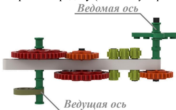
Схема передачи
