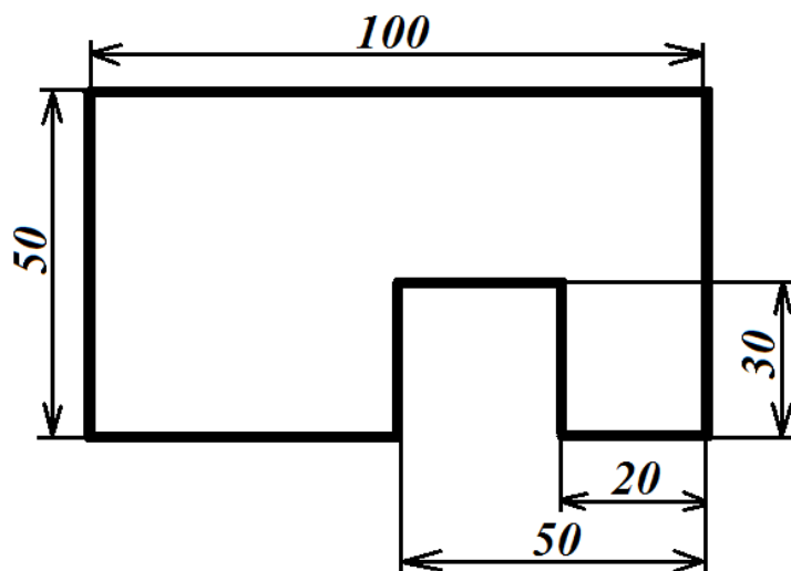
Чертёж детали
